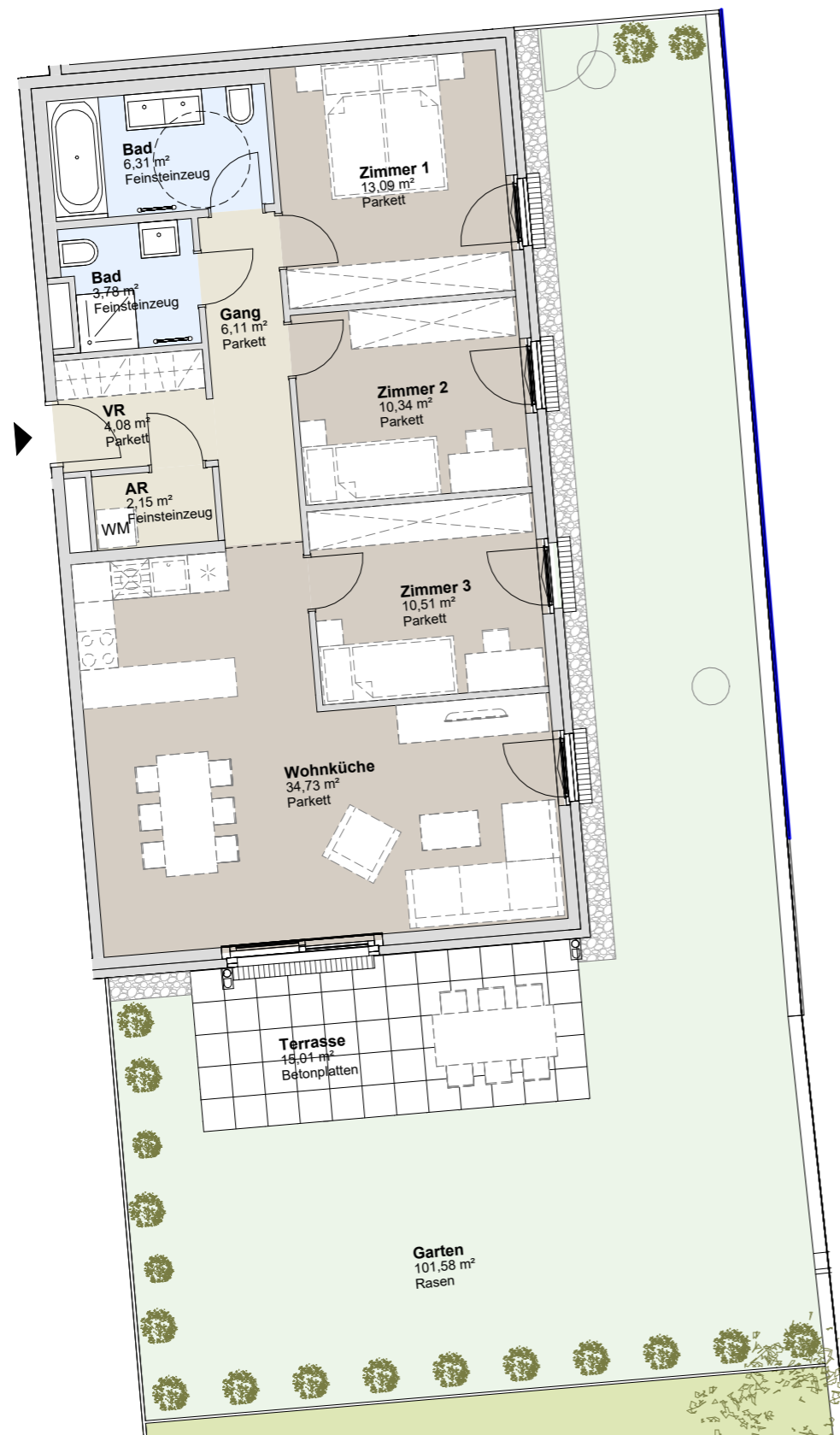
ERDGESCHOSS GARTENBAUKÖRPER
